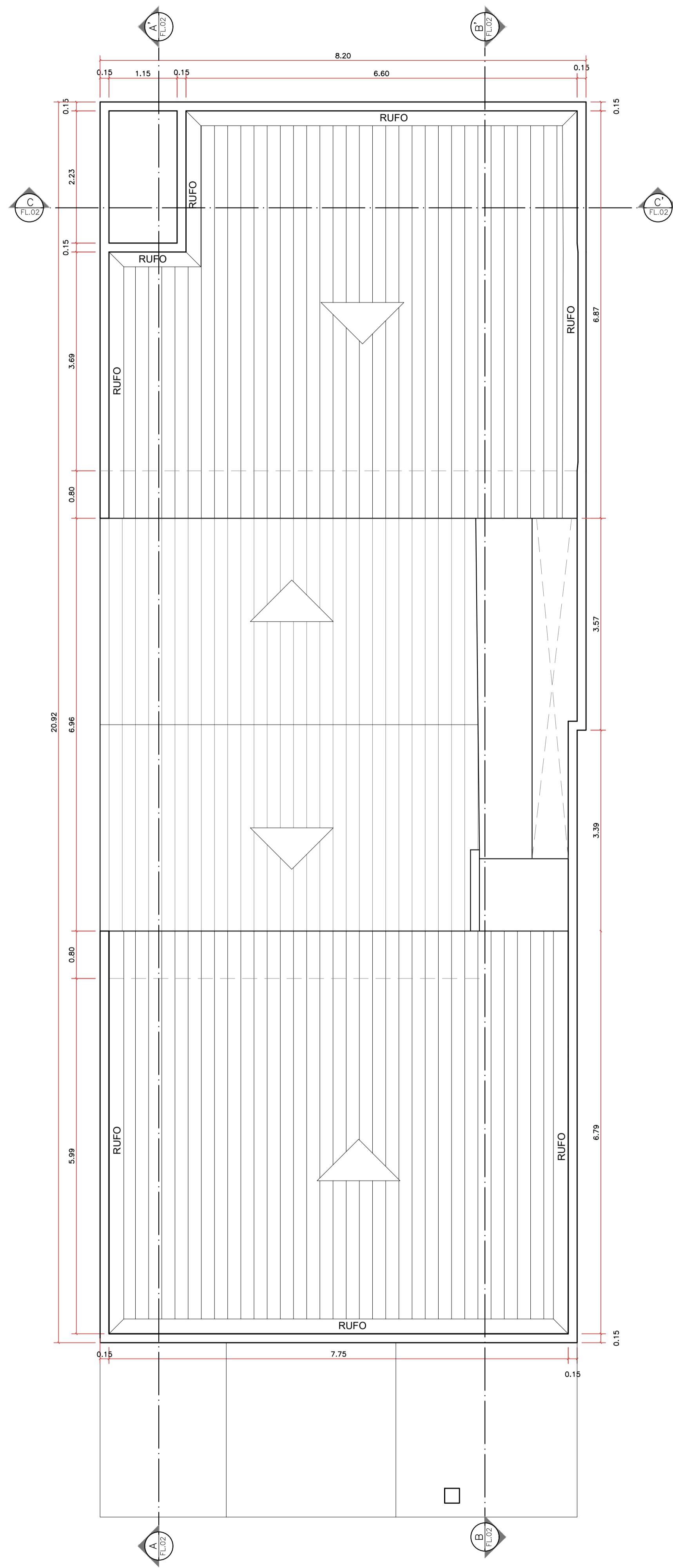
PLANTA DE COBERTA ESC. 1:50
