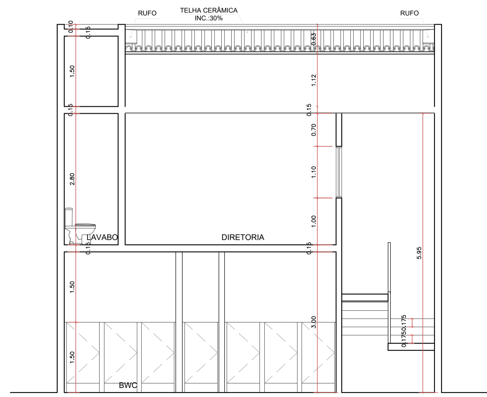
CORTE CC Esc. 1:50
