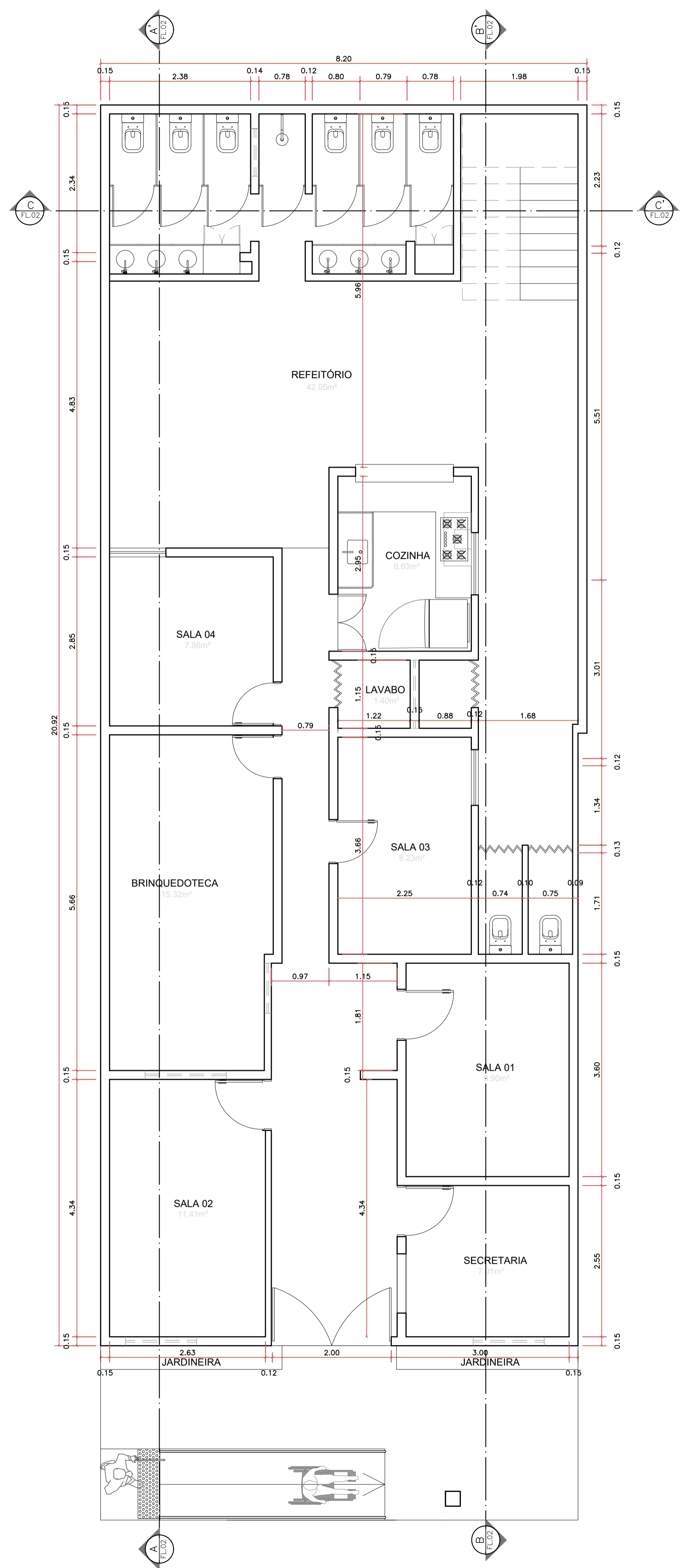
PLANTA BAIXA TÉRREO ESC. 1:50
