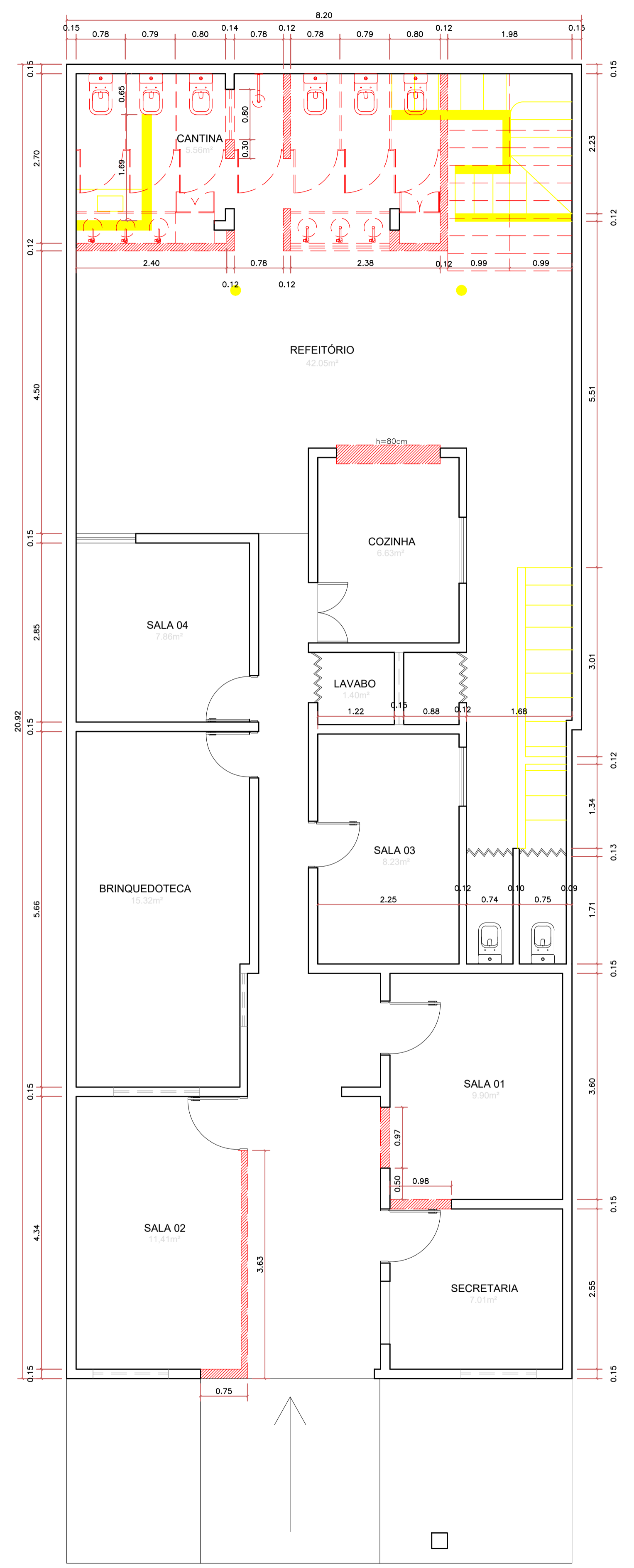
PLANTA BAIXA TÉRREO ESC: 1/50
