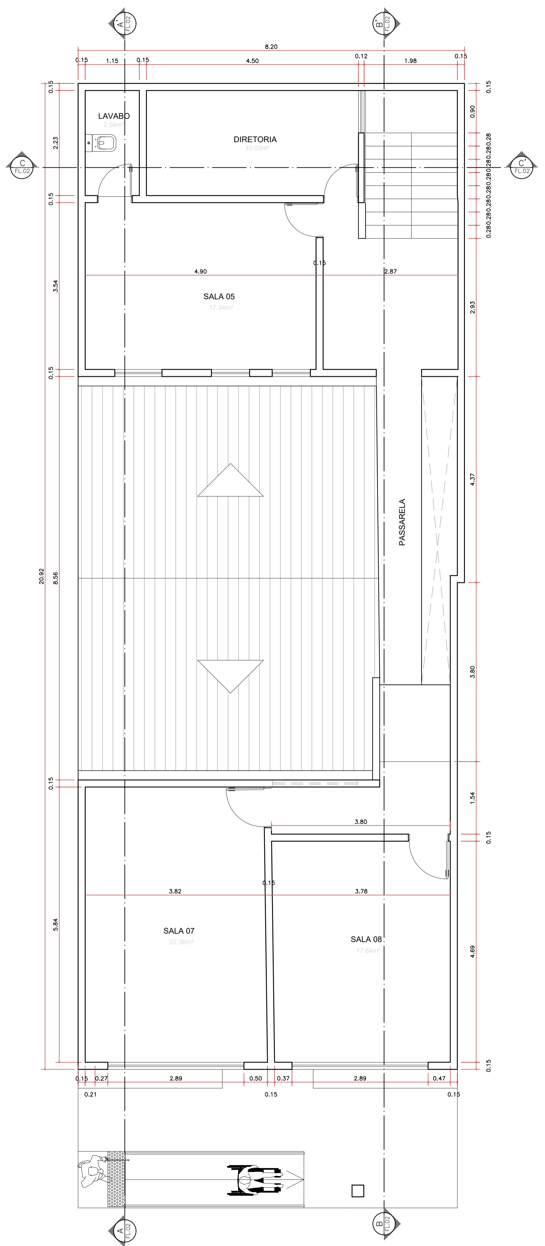
PLANTA BAIXA 1 PAVTO ESC. 1:50
