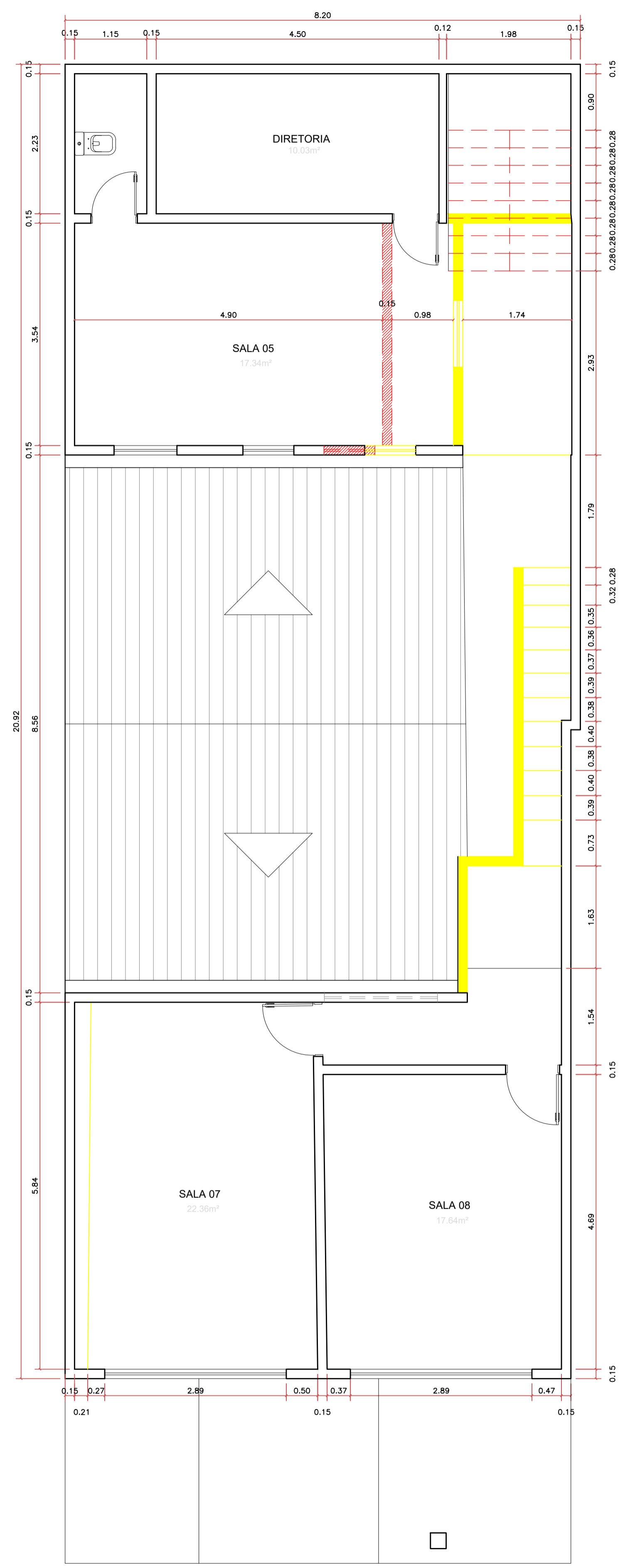
PLANTA BAIXA 1 PAVTO ESC: 1/50
